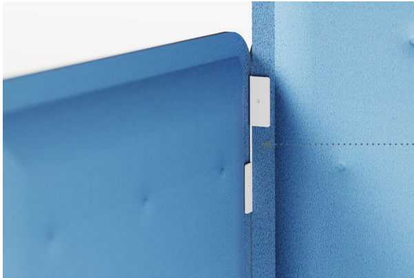
Supporto per la giunzione di due pannelli con lunghezza differente a 90° Sinistro Junction of 2 panels of different sizes 90° LEFT Cod. SFSSDISX
